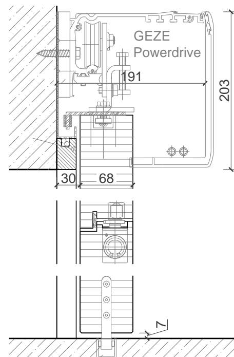
Antrieb und Bodenführung (Vertikalschnitt)
